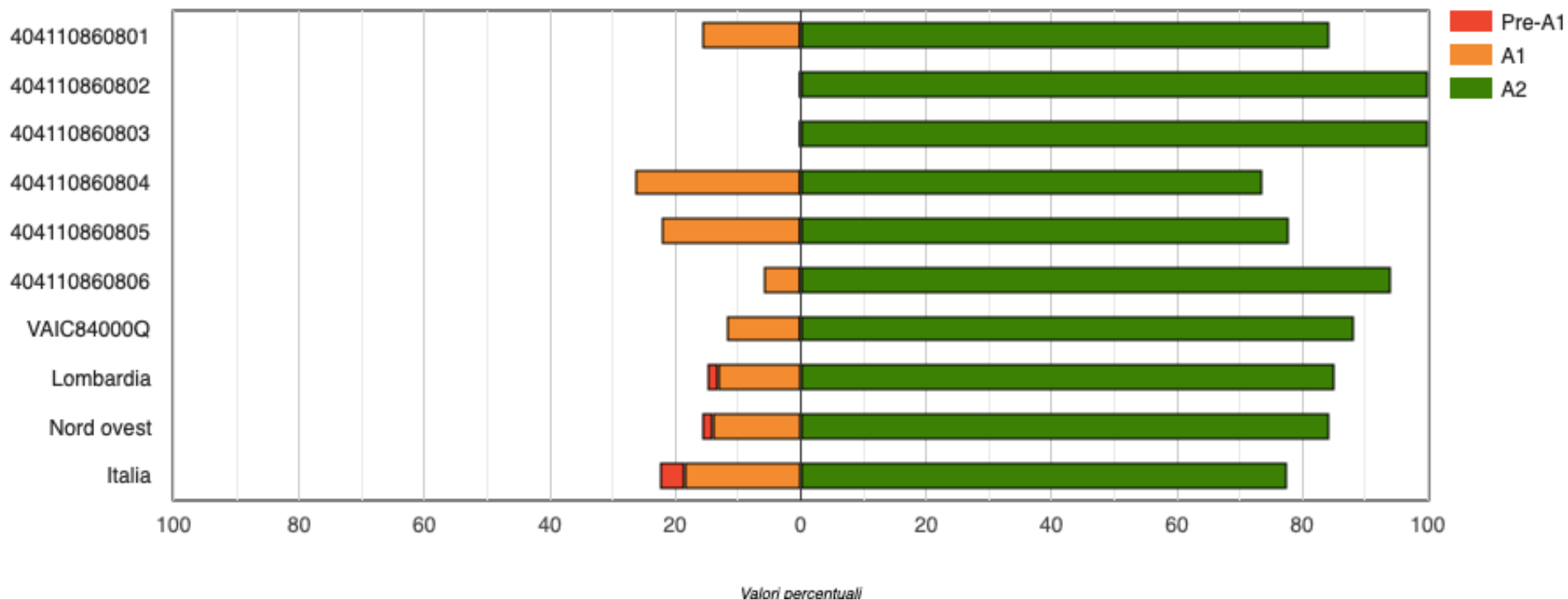
Grafico 2c: VAIC84000Q - Istituto nel suo complesso - Scuola Secondaria di Primo Grado - Classi terze - Prova di Inglese Reading: Distribuzione degli studenti nei livelli di apprendimento
