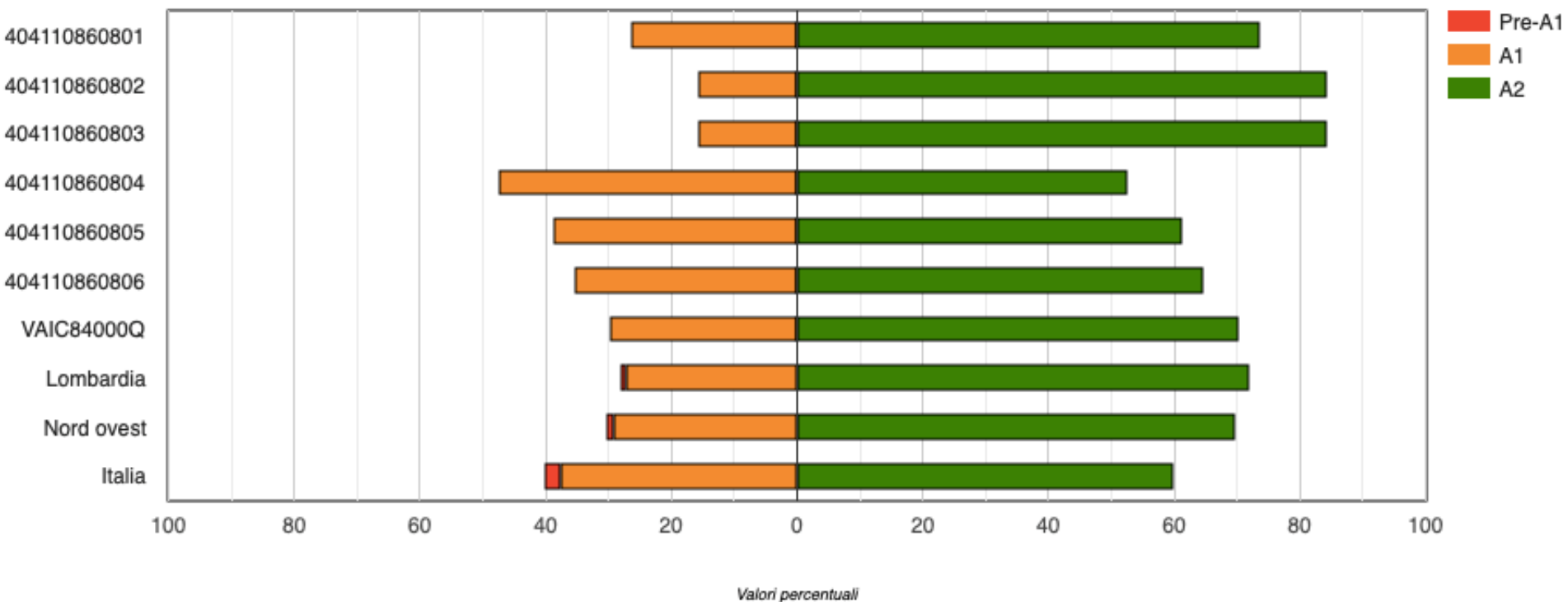
Grafico 2d: VAIC84000Q - Istituto nel suo complesso - Scuola Secondaria di Primo Grado - Classi terze - Prova di Inglese Listening: Distribuzione degli studenti nei livelli di apprendimento
